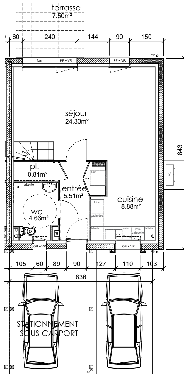
Rez-de-Chaussée
