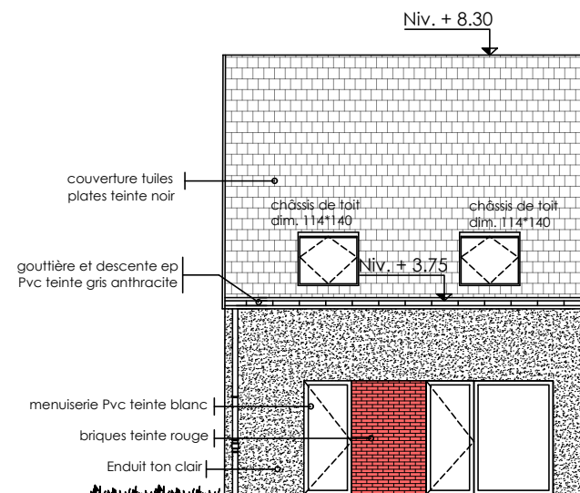
Façade Arrière
